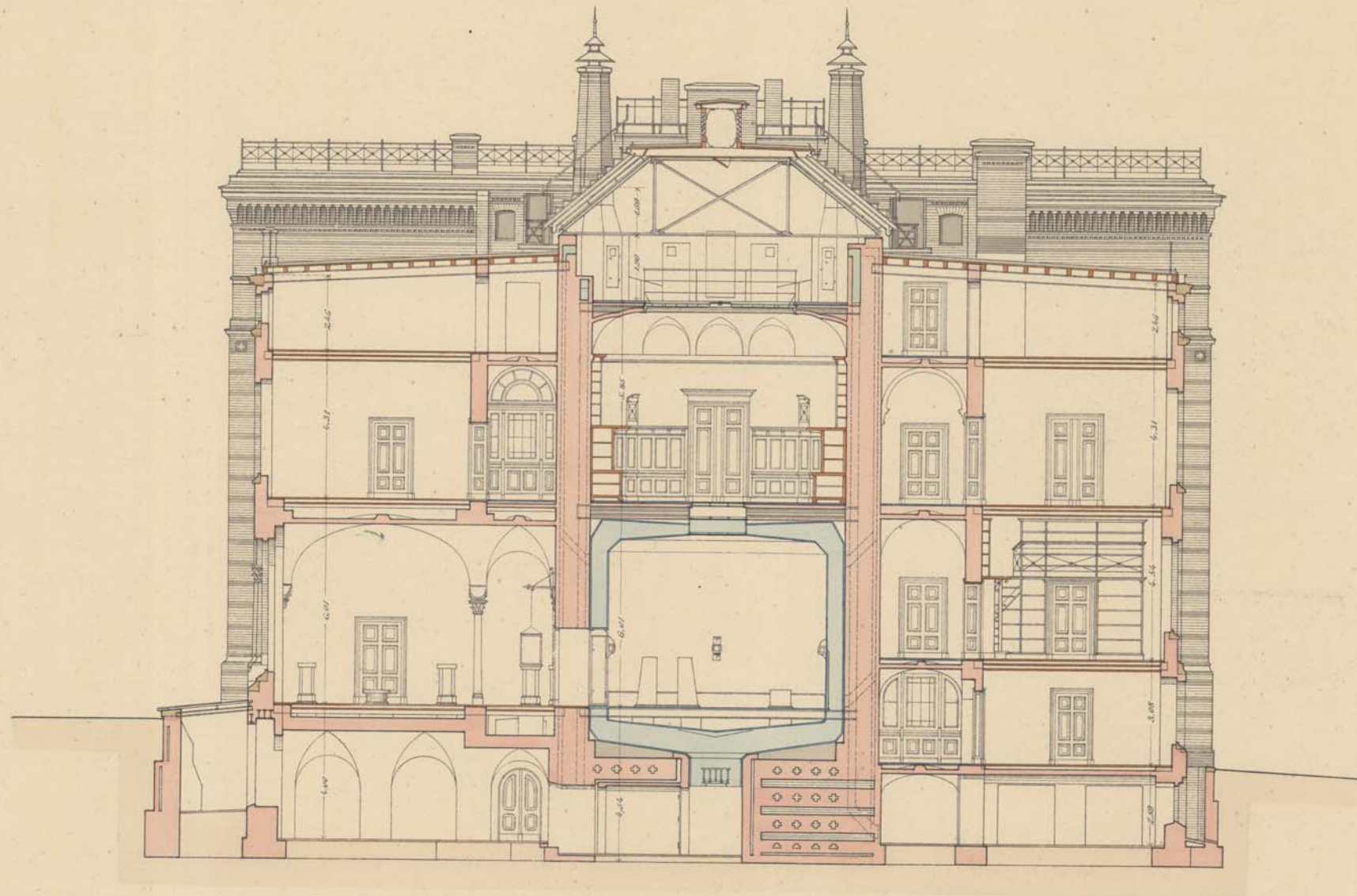
Querschnitt.
