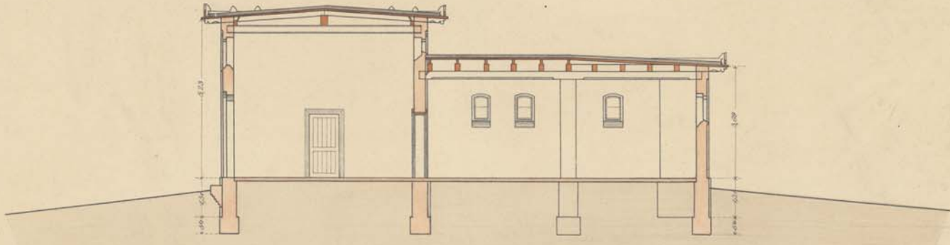
Schnitt A-B.
