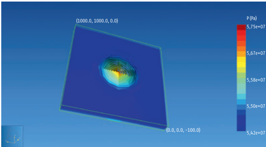
Abb. 5 – Druckverteilung in einem Modellaquifer, in den über eine 100 m lange freie Bohrstrecke über-kritisches CO 2 mit einer Flussrate von 70 kg/s über einen Zeitraum von 70 Tagen injiziert wurde. Der initiale Druck betrug dabei 2 \times 10^7 Pa.
