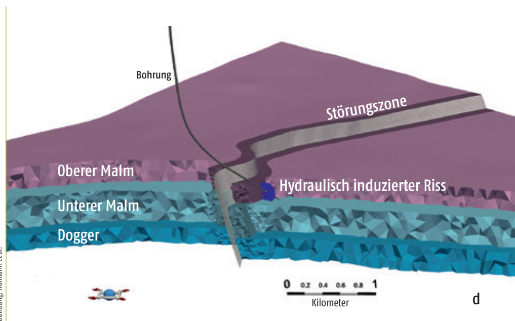
Abb. 4 – Finite-Elemente-Gitter mit den Einheiten Oberer Malm, Unterer Malm und Dogger. Das Szenario enthält eine permeable Störungszone und einen hydraulisch induzierten Riss im Oberen Malm, der die Bohrung mit der Störungszone hydraulisch verbindet.
