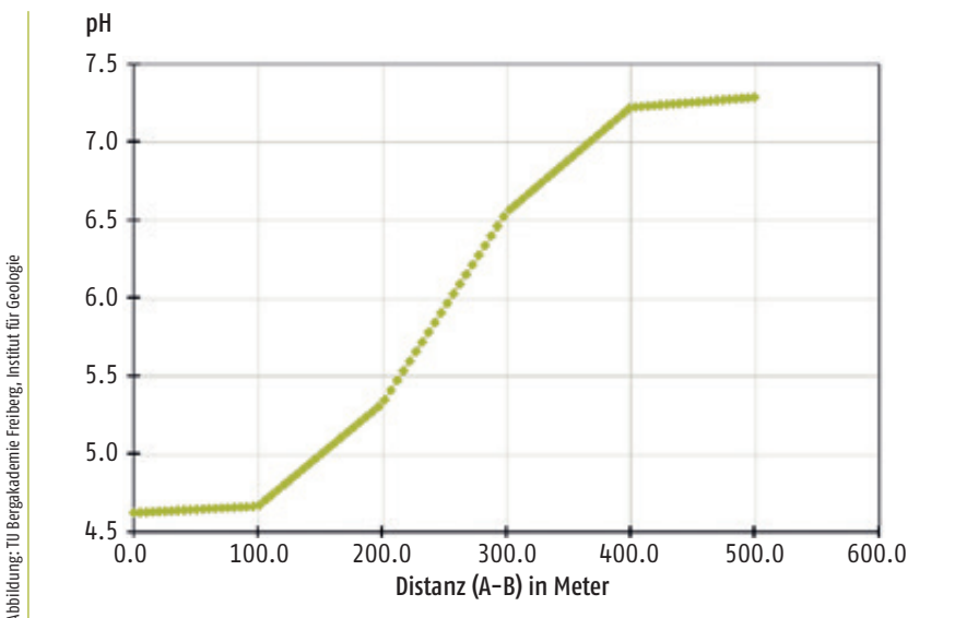
Abb. 6 – Modellerte pH-Werte um das Injektions-Bohrloch nach 70 Tagen
