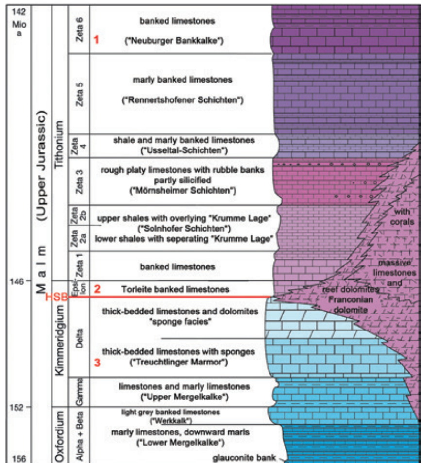
Abb. 2 – Stratigraphie der Schwäbischen Alb des Oberen Jura von Malm Alpha bis Malm Zeta 6 mit Kennzeichnung der Analogaufschlüsse Neuburger Bankkalk (1), Kelheimer Riffkalk (2) und Treuchtlinger Marmor (3). Die hydraulische Stratigraphie-Grenze (HSB) teilt den Malm in einen oberen und einen unteren Teil mit unterschiedlichen hydraulischen und mechanischen Eigenschaften.
