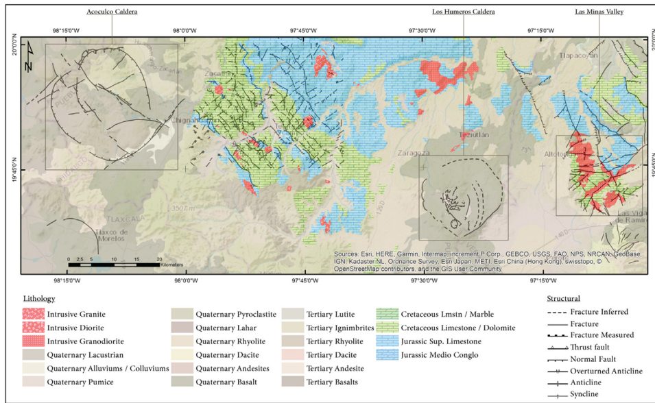
Fig. 8. Geological map of Acozulco – Los Humeros – Las Minas area, modified from (Servicio Geológico Mexicano, 1997, 2002) maps.
