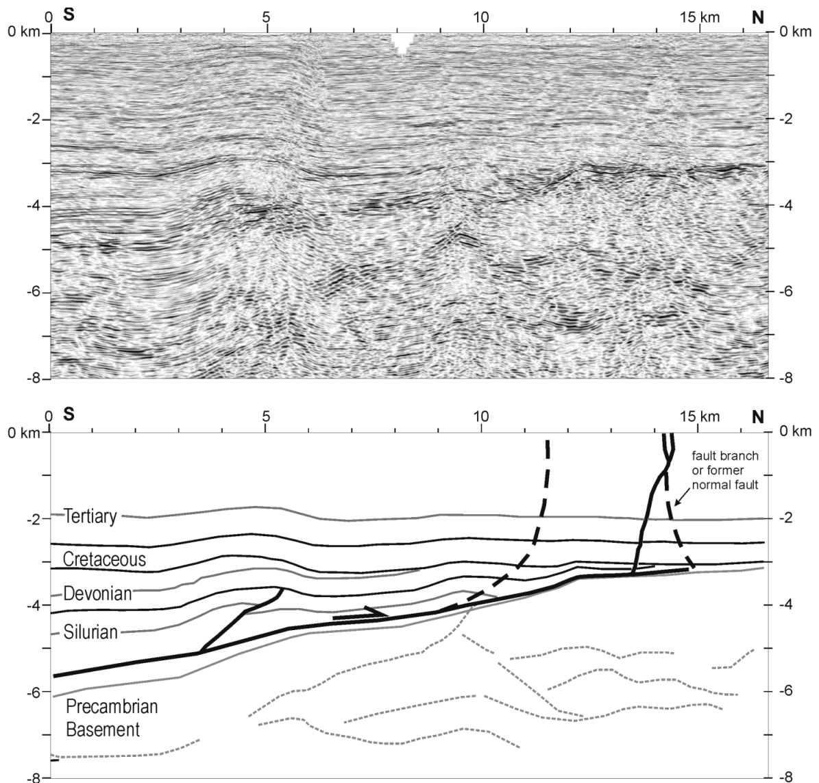
Abb. 4-14 Reflexionsseismisches Profil (oben, zeitmigriert und tiefenkonvertiert, Teilbereich der Linie 6300-31) und Interpretation (rechts, Lage in Abb. 4-2, 4-9). Das Profil zeigt die Faltung über einer Zweigstörung vom Abscherhorizont sowie mehrerer vermutete Störungsspuren eines Blattverschiebungssystems an der nordwestlichen Begrenzung der Boomerang Hills Überschiebungseinheit.
