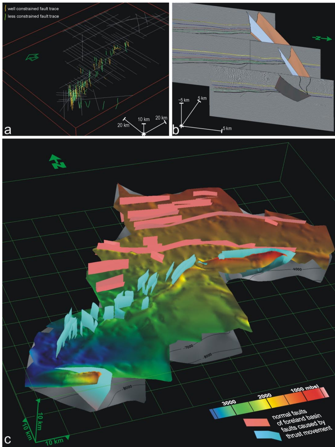
Abb. 5-3 a) gOcad Ansicht der klassifizierten Störungen, hier vereinfacht in zwei Klassen. b) Beispiel von konstruierten Störungsflächen zwischen seismischen Profilen, vgl. Abb.4-15. c) Aus Interpretationen von reflexionsseismischen Profilen konstruiertes Strukturmodell aus Horizonten und Störungen. Oberer Horizont: Tertiärbasis, konturierte Fläche darunter: Grundgebirgsoberfläche, Konturen sind in m unter NN.
