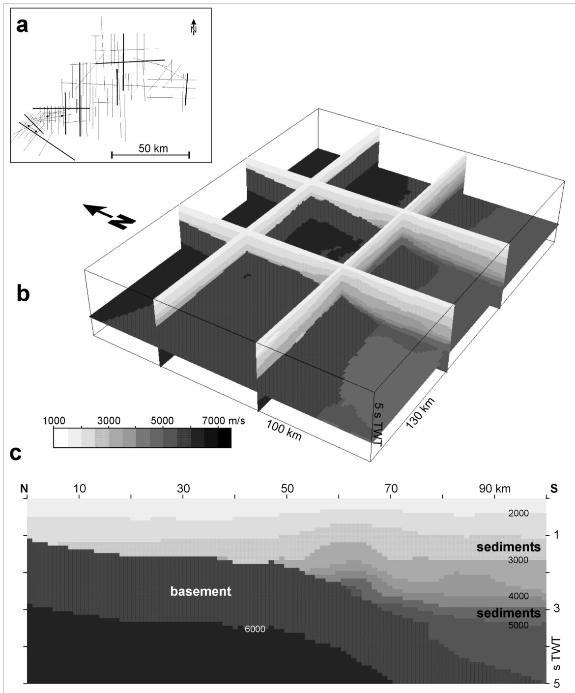
Abb. 3-2 Geschwindigkeitsmodell für Tiefenkonvertierung. a) Position der seismischen Profile für die Intervallgeschwindigkeiten vorliegen (dicke Linien) und der vier verwendeten synthetischen Bohrlochseismogramme (Punkte). b) Perspektivische Ansicht des Geschwindigkeitsmodells mit ausgewählten Schnitten. Die Unterteilung in Deck- und Grundgebirge ist besonders gut im Norden des Modells anhand eines deutlichen Geschwindigkeitssprunges erkennbar. c) Beispielschnitt in N-S Richtung. Sowohl b) als auch c) sind zur Veranschaulichung mit einer diskontinuierlichen Graftonskala dargestellt (500 m/s Intervalle); die Werte im Modell sind tatsächlich kontinuierlich.
