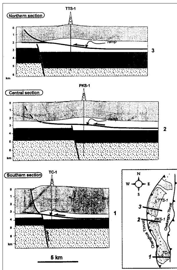
Abb. 6-13 Drei Profile über die Deformationsfront in West Taiwan. Signatur (von oben nach unten): grau = Pleistozän, weiss = Pliozän, dunkelgrau = Miozän, gepunktet: prämiozäne Sedimente. Die Einsatzskizze zeigt die Lage der Profile (Abbildung aus Mouthereau et al., 1999).
