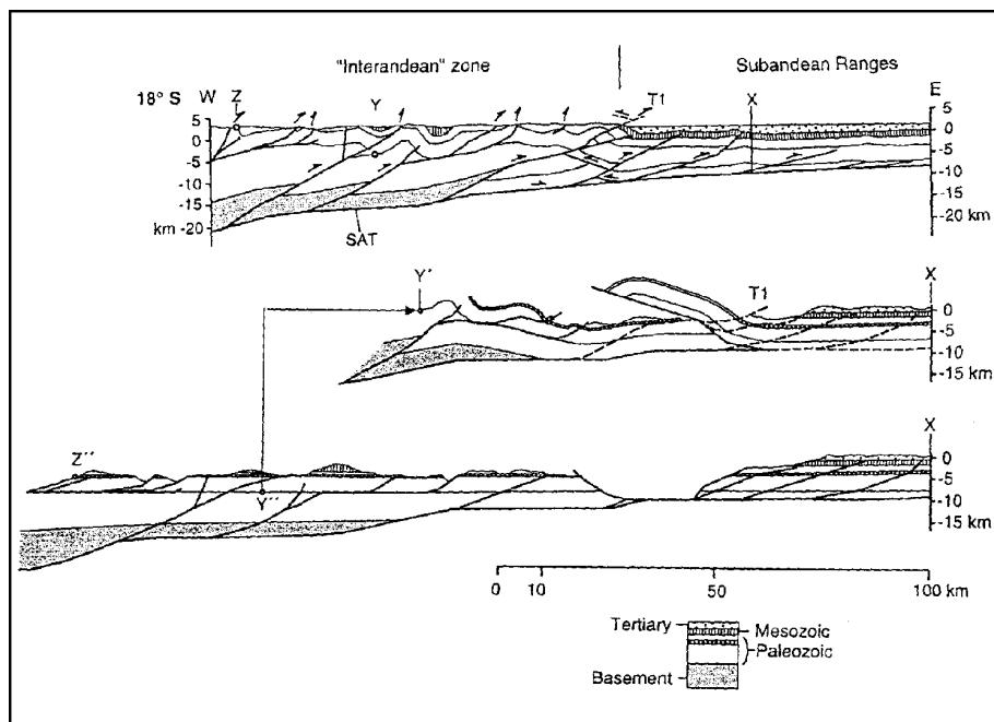
Abb. 6-8 Bilanziertes Profil mit Abwicklung in 2 Inkrementen zur Veranschaulichung, wie strukturell nicht erhaltene Verkürzungsbeträge mittels einer Dreieckszone (erstes Inkrement) im Falten- und Überschiebungsgürtel südlich des Santa Cruz Bogens erklärt werden könnten (aus Kley, 1999). Lage des Profils in Abb. 6-7.
