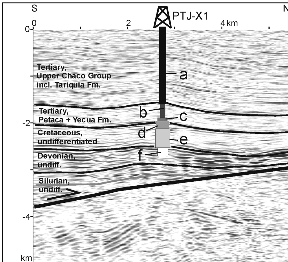
Abb. 3-3 Beispiel eines tiefenkonvertierten seismischen Profils (Teilbereich von Linie 3492-30, Lage in Abb. 3-1). Die Qualität der Konversion kann mit der stratigraphischen Information der Bohrung PTJ-X1 kontrolliert werden (a: Tertiär, Obere Chaco Gruppe inkl. Tariquia Formation (Fm.); b: Tertiär, Yecua Fm.; c: Tertiär, Petaca Fm., d: Kreide, Yantata Fm.; e: Kreide, Ichoa Fm.; f: Devon, nicht differenziert).
