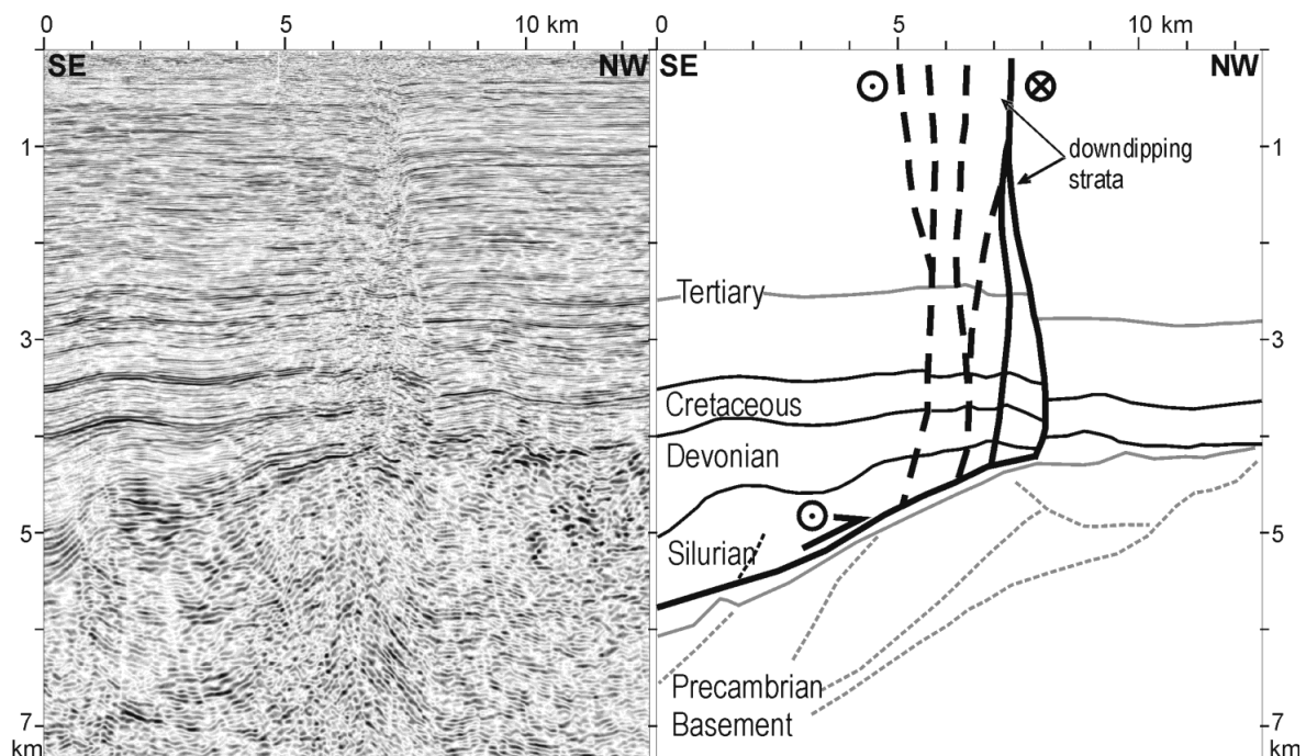
Abb. 4-11 Reflexionsseismisches Profil (links, zeitmigriert und tiefenkonvertiert, Teilbereich der Linie 1052-22) und Interpretation (rechts), die das Transferstörungssystem am westlichen Ende der Boomerang Hills Überschiebungseinheit zeigt (Profil zweifach überhöht, Lage in Abb. 4-2, 4-9).
