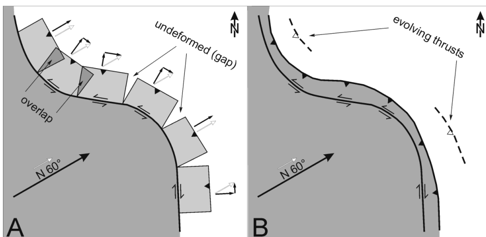
Abb. 6-5 Skizze zur Verdeutlichung der räumlichen Probleme des Materialtransfers bei frontaler Akkretion in gebogenen Falten- und Überschiebungsgürteln. A) Initiales Stadium der Bildung neuer Überschiebungseinheiten. Die neuen Überschiebungen brechen parallel zu den bereits akkretierten Körpern (dunkelgrau). B) Theoretisch resultierende Form der neuen Deformationsfront.
