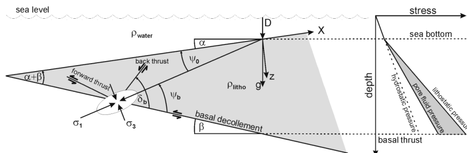
Abb. 5-11 Schematisches Profil durch einen submarinen Deckenkeil zur Veranschaulichung der geometrischen Größen zur Berechnung von kritischen Keilmodellen. Die Parameter sind im Text erläutert. Rechts: In Grau dargestellt ist der Bereich der effektiven Spannung, verursacht durch einen Porenflüssigkeitsdruckgradienten, der über dem hydrostatischen Gradienten liegt (modifiziert nach Dahlen und Suppe, 1988).
