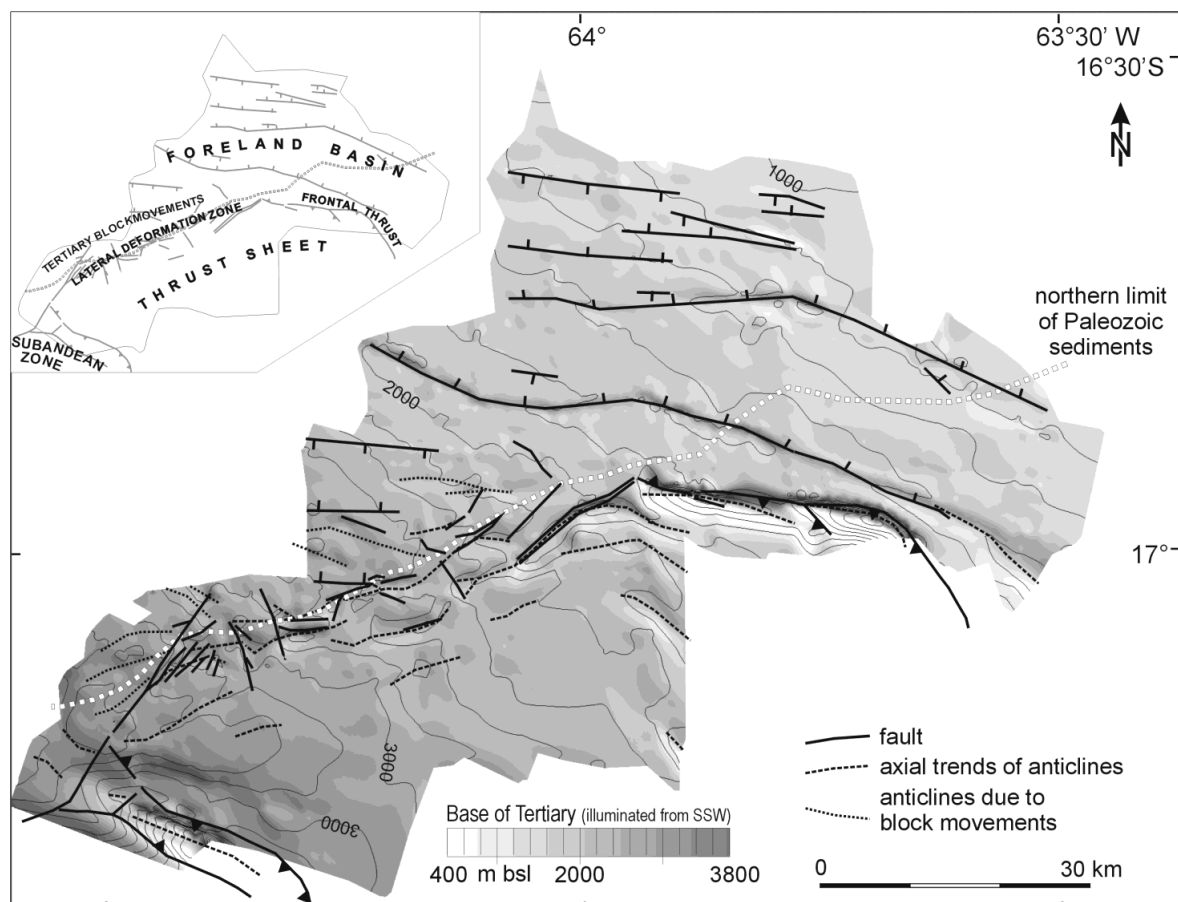
Abb. 4-5 Strukturkarte der Tertiärbasis mit Fläche der Tertiärbasis, basierend auf den Interpretationen reflexionsseismischer Profile. Die Karte zeigt den Übergang vom Falten- und Überschiebungsgürtel der Subandinen Zone zum Andenvorland nordwestlich von Santa Cruz, Bolivien. Der südliche Teil der Karte zeigt Strukturen der konvergenten andinen Deformation mit der jungen, sich entwickelnden Boomerang Hills Überschiebungseinheit. Die im Text verwendeten Strukturdomänen sind in dem Karteneinsatz verzeichnet.
