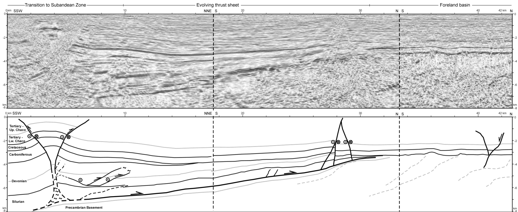
Abb. 4-1 Zusammengesetztes seismisches Profil (oben, zeitmigriert und tiefenkonvertiert) und Interpretation (unten), welches die Struktur von der Spitze der Subandinen Zone bis ins Andenvorland zeigt (siehe Abb. 4-2, bzw. 4-9 für Position). Das Profil basiert auf Teilen der Linien 3532-30, 3514-30 und 3512-31p (siehe Abb. 3-1).
