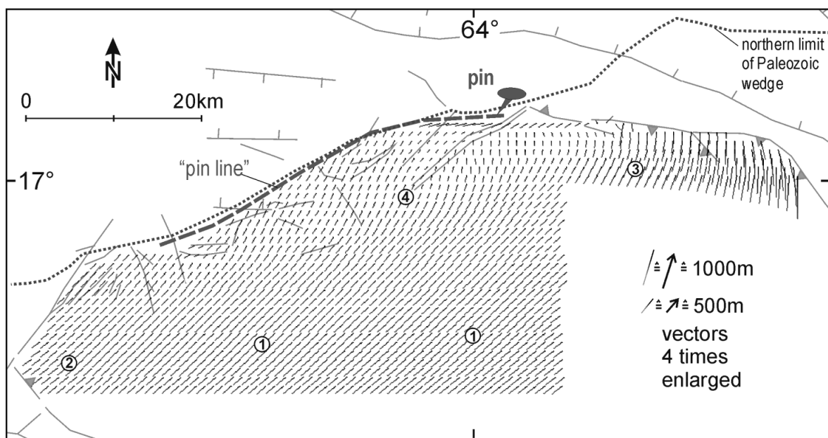
Abb. 5-9 Faltenbezogene Partikelpfade in der jungen, sich entwickelnden Boomerang Hills Überschiebungseinheit. Das Verschiebungsfeld basiert auf der Retrodeformation der verfalteten Tertiärbasis mit der UNFOLD Methode (Gratier et al. 1991) und einem darauf aufbauenden erweiterten Ansatz. Die Zahlen 1-4 kennzeichnen Punkte, die im Text besprochen werden.
