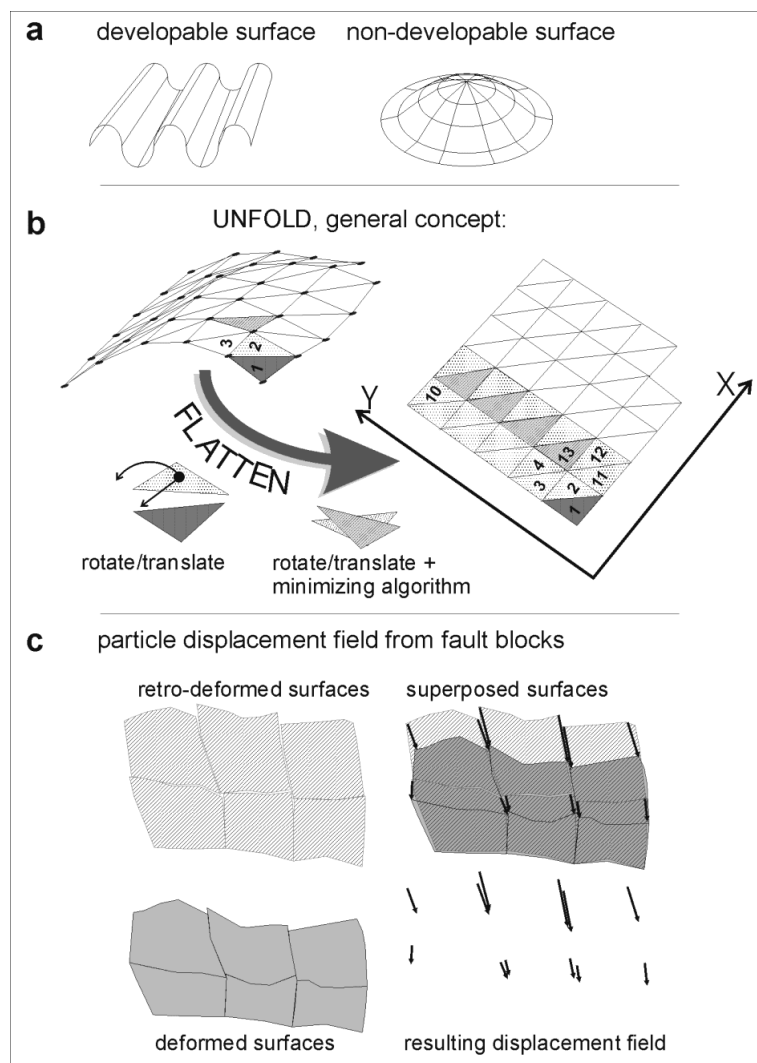
Abb. 5-6 Konzept der Restaurierung verfalteter Flächen.
