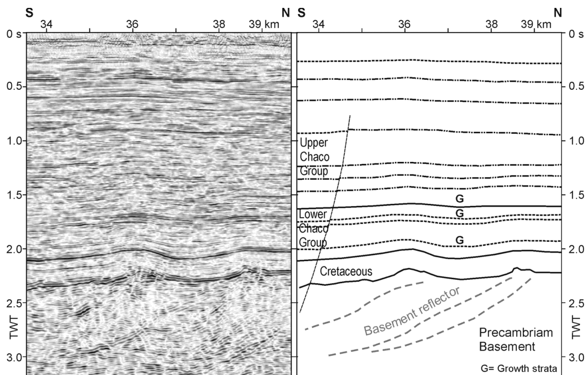
Abb. 4-6 Reflexionsseismisches Profil (links, Ausschnitt des Profils in Abb. 4-1) und Interpretation (rechts) zur Verdeutlichung der syntektonischen Sedimentation in Zusammenhang mit tertiären Grundgebirgsbewegungen im Vorland der Zentralen Anden bei 17° S zwischen 64-64.5°W. Überhöhung ca. 1.7 bei 2 s TWT.
