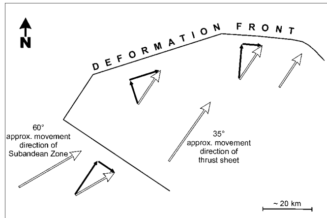
Abb. 6-4 Vereinfachte Skizze zur Erläuterung der Verformungsaufteilung am rückwärtigen Ende und an der Deformationsfront der Boomerang Hills Überschiebungseinheit.
