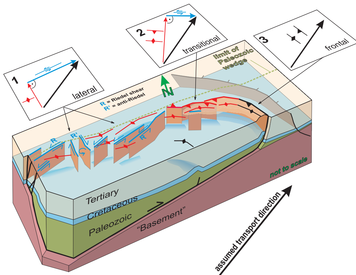
Abb. 5-5 Blockbild mit vereinfachten Strukturen zur Verdeutlichung der Verformungsaufteilung an der Deformationsfront der Boomerang Hills Überschiebungseinheit.
