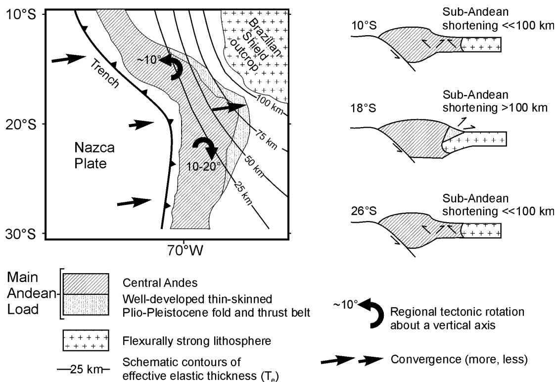
Abb. 2-7 Schematische Abbildung zur Illustration des Zusammenhangs zwischen effektiver elastischer Plattendicke ( T_e ) und dem Deformationsmodus im östlichen backarc der Zentralen Anden (nach Watts et al., 1995).
