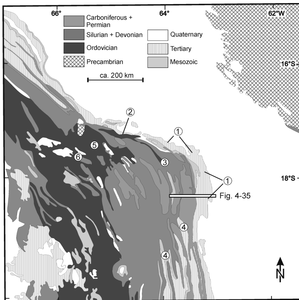
Abb. 6-7 Geologische Karte der östlichen zentralen Anden im Bereich des Andenkniekes (Basierend auf einer vereinfachten Version der geologischen Karte von Bolivien nach YPFB und Sergeomin, 1996). Die Zahlen 1-5 kennzeichnen Punkte, die im Text besprochen werden.
