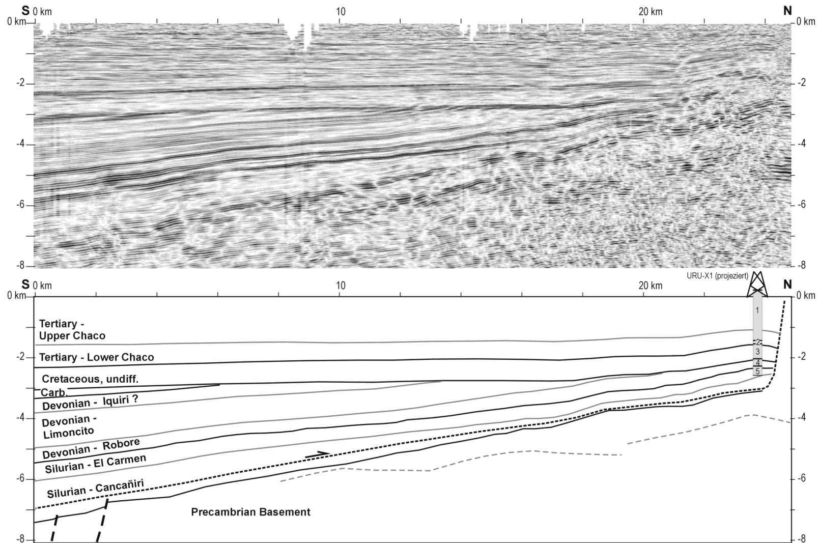
Abb. 2-10 Reflexionsseismisches Profil (oben, zeitmigriert und tiefenkonvertiert) und Interpretation (unten) zur Veranschaulichung der Abbildungseigenschaften der kartierten Gruppen und Formationen (Teilbereich von Linie 3482-26, Lage siehe Abb. 3-1). Die Bohrung URU-X1 ist ca. 3 km projiziert und auf ca. 240 m NN höhenkorrigiert. 1: Obere Chaco Gruppe und Tariquia Formation, 2: Yecua und Petaca Formationen, 3: Yantata und Ichoa Formationen, 4: Devon, undifferenziert, 5: Silur, undifferenziert; Carb. = Karbon, undifferenziert.
