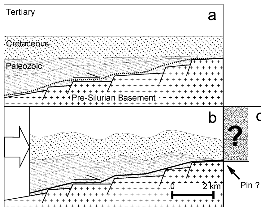
Abb. 2-8 Von Welsink et al. (1995) vorgeschlagenes Modell zur Erklärung der Faltengeometrien im Bereich der Boomerang Hills Region durch passives Falten der abgescherten Sedimente über Stufen im Abscherhorizont. a) Ausgangssituation, b) mit dem Programm „Thrust Belt“ vorwärtsmodellierter Faltenbau (modifiziert nach Welsink et al., 1995), c) die graue Fläche repräsentiert die im Vorwärtsmodell (a, b) theoretisch erzeugte, aber nicht berücksichtigte horizontale Exzessfläche, die auf eine nicht vorhandene fixierte Referenzlinie zurückzuführen ist. Die theoretisch erzeugte vertikale Exzessfläche ist nicht dargestellt.
