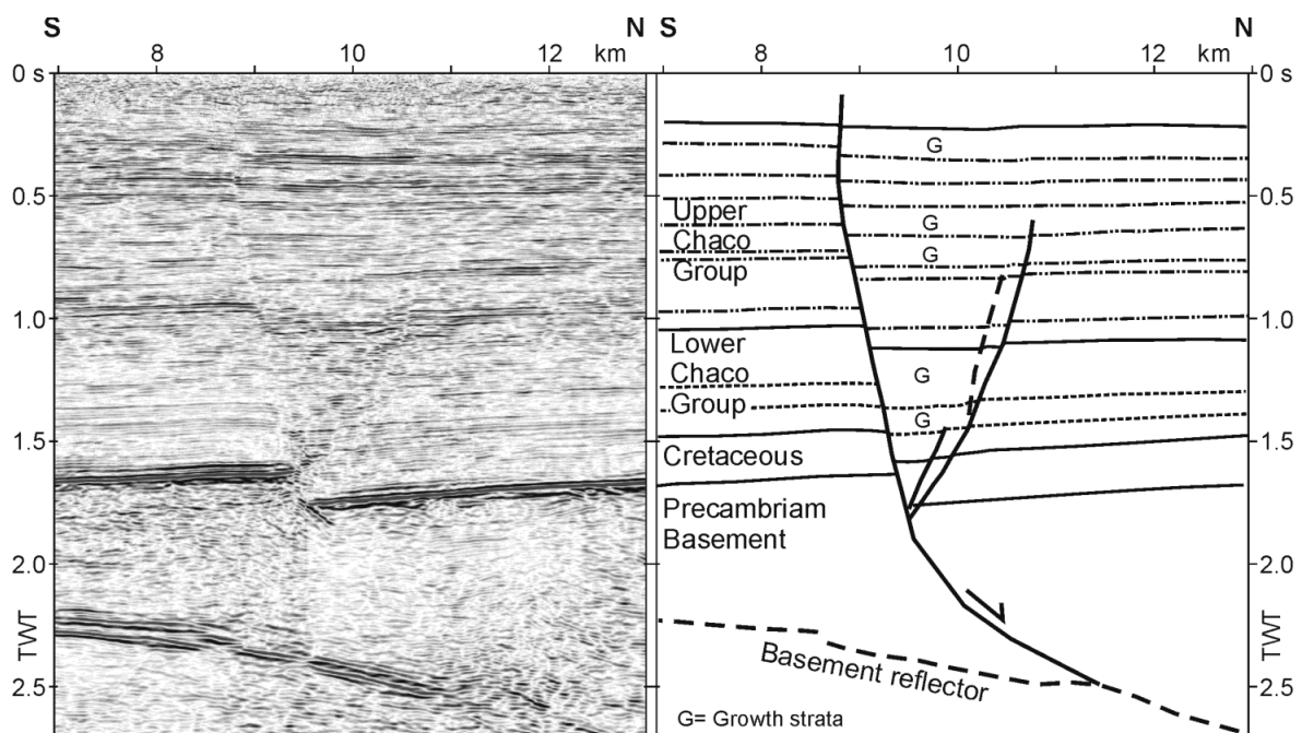
Abb. 4-7 Reflexionsseismisches Profil (links, Ausschnitt aus Abb. 4-4) und Interpretation (rechts) zur Verdeutlichung der syntektonischen Sedimentation an tertiären Abschiebungen im Vorland der Zentralen Anden zwischen 16.5° und 17° S. Überhöhung ca. 1.8 bei 1.7 s TWT.
