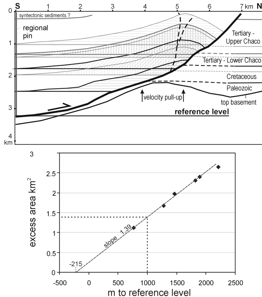
Abb. 5-1 Geometrische Analyse des Falten-Störungssystems an der frontalen Spitze der Boomerang Hills Überschiebungseinheit (aus Abb. 4-10) zur Bestimmung der Abscherhorizonttiefe und des Versatzes. Der Schnittpunkt der Regressionsgeraden mit der Abszisse ergibt die Tiefe zum Abscherhorizont (-215 m unter dem Referenzhorizont). Die Steigung entspricht dem Versatz auf dem Abscherhorizont (1390 m; Methode nach Epard und Groshong, 1993)
