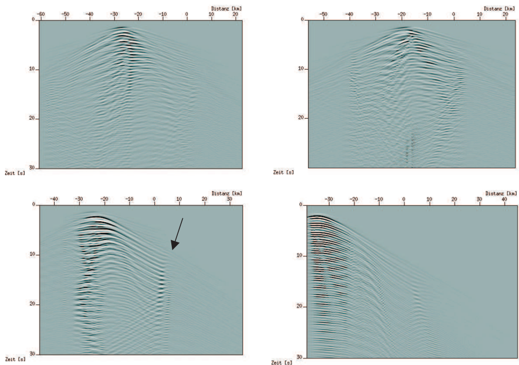
Abbildung 4.18: EW-Komponenten der Bodenschwingungsgeschwindigkeit (in einheitlicher Skalierung) für die 4 Profile aus Abbildung 4.17 (in derselben Anordnung). Der Referenzpunkt für die Distanzskalierung befindet sich am Kreuzungspunkt der Profile (+ in Abbildung 4.17).
