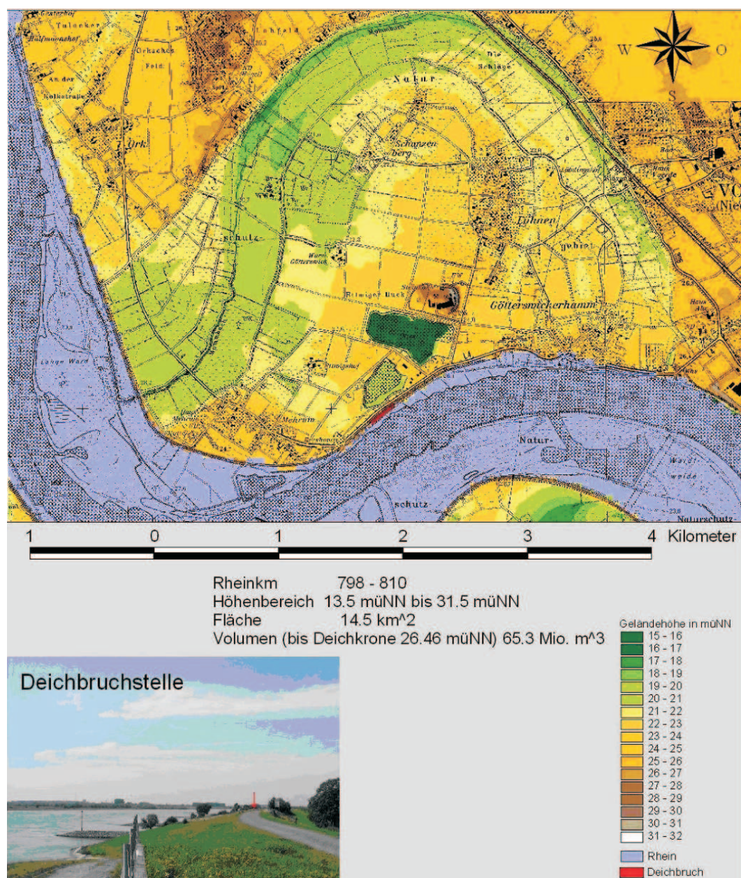
Abbildung 2.25: Überflutungsgebiet mit Deichbruchstelle (Kreis)
