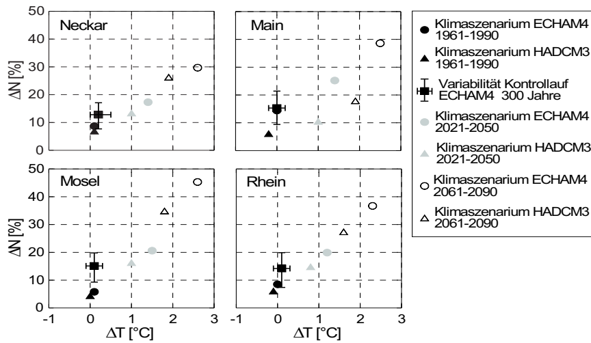
Abbildung 2.11: Abweichungen von den aus Stationsmessungen 1961-1990 bestimmten Gebietsmitteln des Niederschlags N und der Temperatur T, dargestellt für drei Teilgebiete sowie das gesamte Rhein-Einzugsgebiet zwischen den Pegeln Maxau und Köln. Die Fehlerbalken um die jeweiligen Daten des Kontrolllaufes geben die gesamte Variationsbreite 30-jähriger Mittelwerte über den Simulationszeitraum von 300 Jahren wieder.
