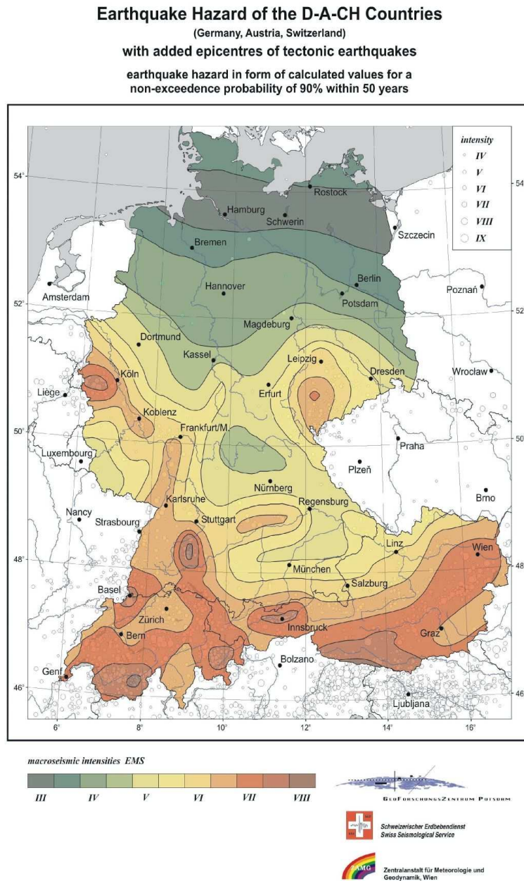
Abbildung 4.44: Erdbebengefährdung für die D-A-CH Staaten (Grünthal et al, 1998)
