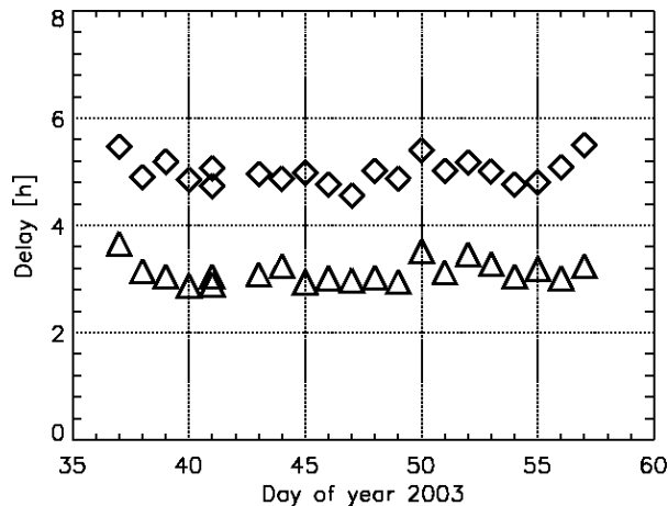
Abbildung 13: Durchschnittliche Verzögerung zwischen Messung und Bereitstellung am Datenzentrum (ISDC) von atmosphärischen Phasenwegverlängerungen für die operationelle Near-Real-Time Datenprozessierung seit dem 6. Februar 2003 (Karas). Die Dreiecke zeigen die minimale Verzögerung pro Tag.
