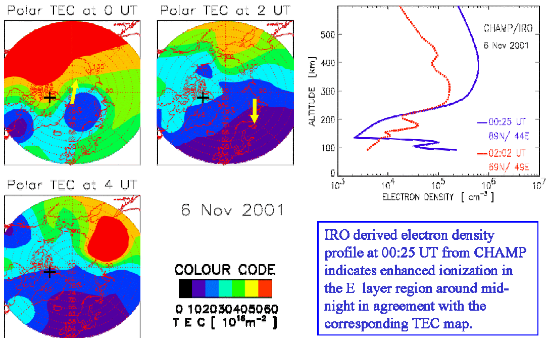
Abbildung 25: Koordinierte IRO-Messungen der vertikalen Elektronendichte mit bodengestützten TEC-Messungen während des Space-Weather-Ereignisses am 6./7. November 2001. Die Ergebnisse ergänzen einander in der physikalischen Aussage (vgl. Jakowski et al., 2003).
