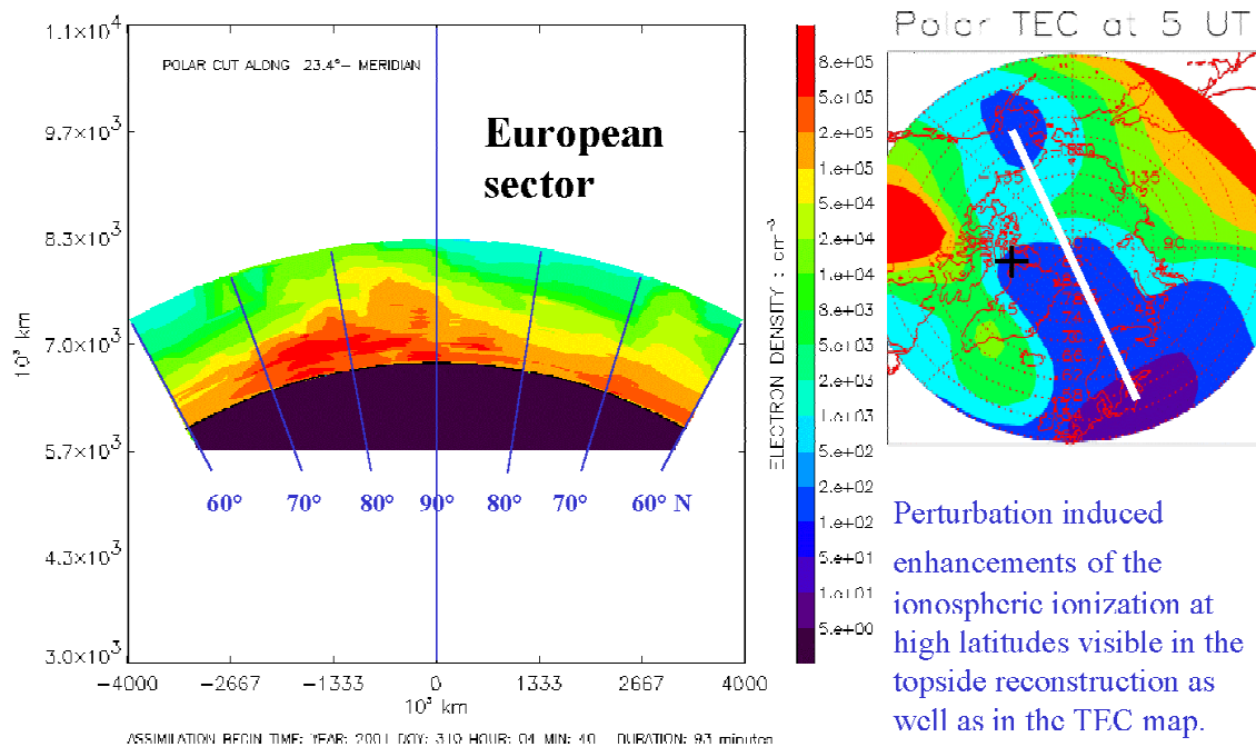
Abbildung 26: Koordinierte 2D-Rekonstruktion der vertikalen Elektronendichte mit bodengestützten TEC-Messungen während des Space-Weather-Ereignisses am 6./7. November 2001. Die TEC-Karte zeigt ebenfalls die Schnittebene der Rekonstruktion. Die Ergebnisse ergänzen einander in der physikalischen Aussage.
