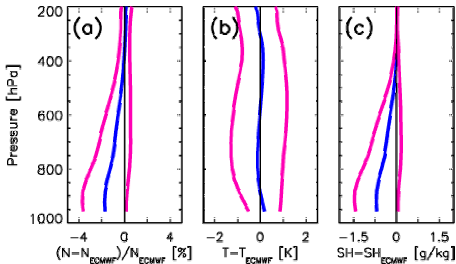
Abbildung 9: Ergebnisse der operationellen Prozessierung mit der Implementierung eines 1D-Var Verfahrens zur Ableitung von Temperatur- und Wasserdampfprofilen aus GPS-Radio-Okkultationsdaten. Die Abbildung zeigt einen Vergleich der abgeleiteten Temperaturen und spezifischen Feuchte mit ECMWF-Daten.
