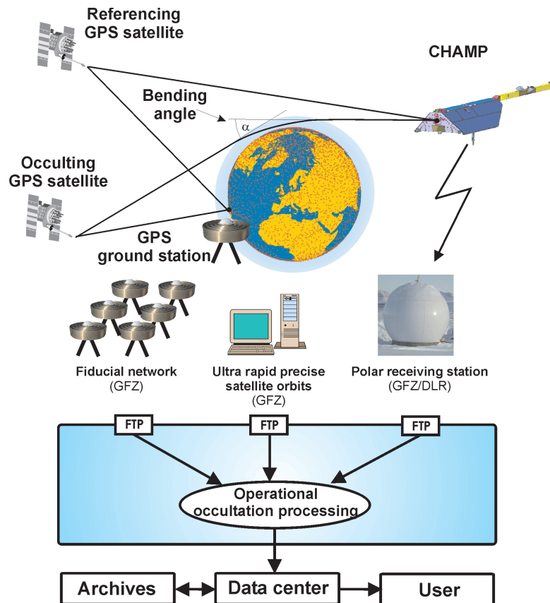
Abbildung 6: Im Rahmen von GASP installierte Infrastruktur zur operationellen Prozessierung und Bereitstellung von GPS-Okkultationsdaten bzw. Analyseregebnissen der CHAMP-Satellitenmission.
