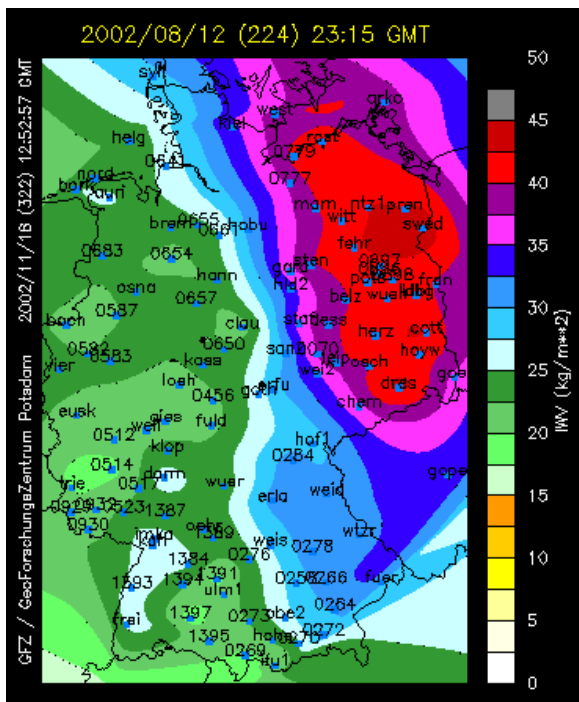
Abbildung 2: Wasserdampffeld über Deutschland mit extremen Werten im östlichen Bereich zur Zeit der Flutkatastrophe an der Elbe (12. August 2002)
