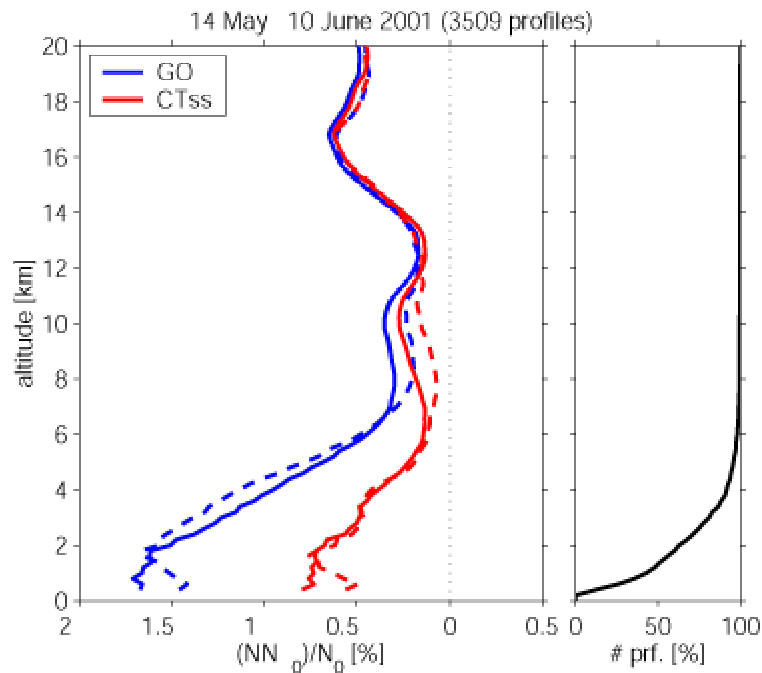
Abbildung 10: Statistischer Vergleich von ~3.500 vertikalen Refraktivitätsprofilen, abgeleitet aus CHAMP-Messungen 2001, mit Ergebnissen von meteorologischen Analysen von ECMWF (durchgezogene Linie: gesamter Datensatz; gestrichelte Linie: Messungen auf der Nordhemisphäre). Die Anwendung der CTss Methode bringt eine deutliche Reduzierung negativen Refraktivitätsbias gegenüber der Anwendung der geometrischen Optik (GO).
