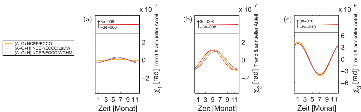
Abbildung 6.10: Einfluss der kontinentalen Wasserspeicherung auf die annuellen \chi -Funktionen im Untersuchungszeitraum 1993–2006. Zum Vergleich sind die summierten geophysikalischen Anregungen (AAM, OAM und HAM) den atmosphärisch-ozeanischen \chi -Funktionen am Beispiel der Modellkombination NCEP/ECCO gegenübergestellt. In (a, b) sind die äquatorialen \chi -Funktionen und in (c) ist \chi_3 abgebildet.
