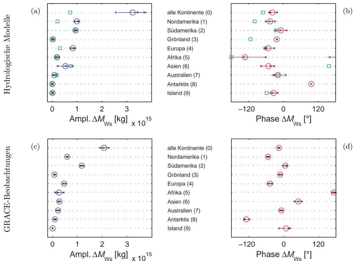
Abbildung 5.9: Analyse des annualen hydrologischen Massenumsatzes und der Einfluss der einzelnen Kontinente auf die Gesamtvariation von \Delta M_{W_s} . In (a, c) sind die Amplituden und in (b, d) sind die Phasen der angepassten trendbereinigten Sinusschwingungen bezogen auf den 1. Januar dargestellt (x). Neben den Mittelwerten für Amplitude und Phase (blaue und rote Kreise) sind die jeweiligen Standardabweichungen als horizontale Fehlerbalken abgebildet. Dabei wurden in (a, b) die Modelle LaDW, WGHM und GLDAS für den Untersuchungszeitraum 1992–2006 miteinander in Beziehung gesetzt. Aufgrund der starken Abweichungen ist H96 (grüne Quadrate) nicht in die Berechnung der mittleren annualen Schwingungen eingegangen. Die aus den Schwerfeldlösungen des GFZ, CSR und CNES abgeleiteten Massenvariationen der Jahre 2002–2006 sind in (c, d) gegenübergestellt.
