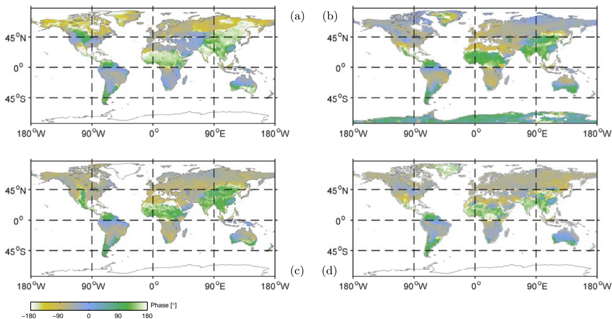
Abbildung 5.2: Phasenwinkel des annualen Signalanteils der kontinentalen Wasserspeicherung in (a) H96, (b) LaDW, (c) WGHM und (d) GLDAS. Die ausgleichende Sinusfunktion pro Gitterzelle bezieht sich für die Modelle (a, b, c) mit 0° Phasenverschiebung auf den 1. Januar 1992, für (d) auf den 1. Januar 2002.
