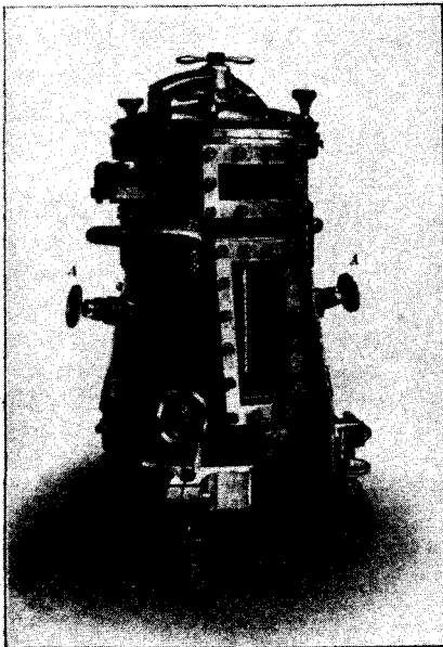
Abb. 3: Der im Geodätischen Institut Potsdam gebaute Pendelapparat der Deutschen Südpolarexpedition.
