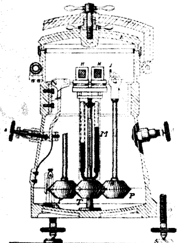
Abb. 3: Der im Geodätischen Institut Potsdam gebaute Pendelapparat der Deutschen Südpolarexpedition.
